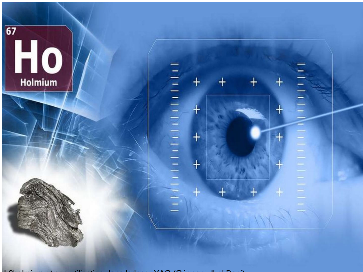
L'holmium et son utilisation dans le laser YAG (Géoparc Jbel Bani)
