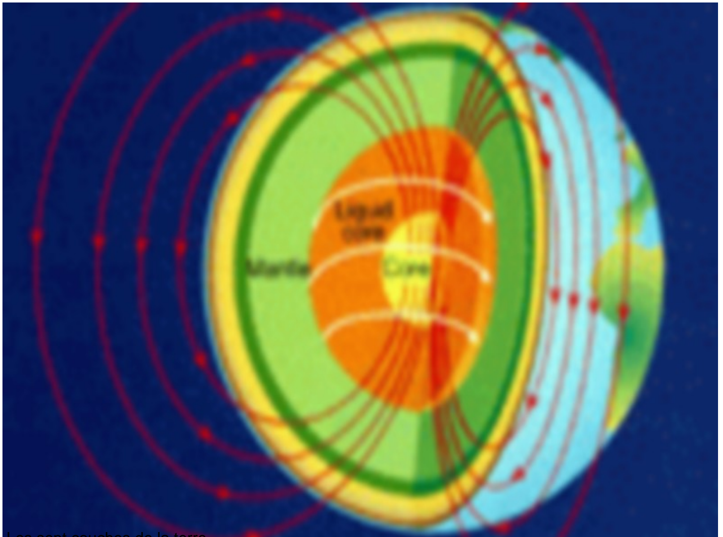
Les sept couches de la terre
